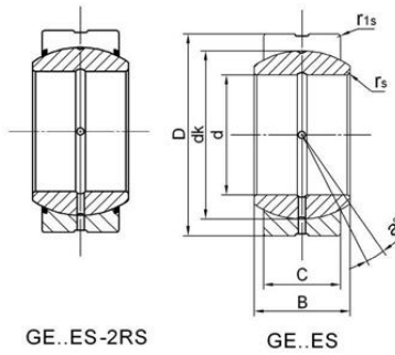
GE..ES-2RS
